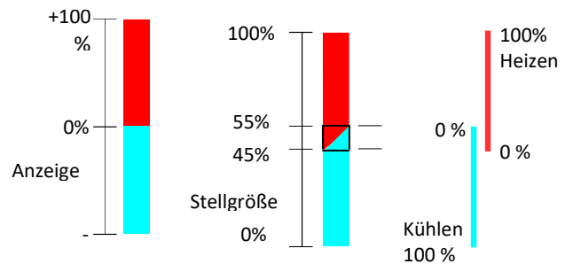
Schaltabstand = -10 % gleichzeitig Heizen und Kühlen
