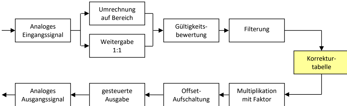
Bild 1: Funktionsschema des Istwertblockes
