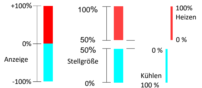
Schaltabstand = +10 % weder Heizen noch Kühlen
