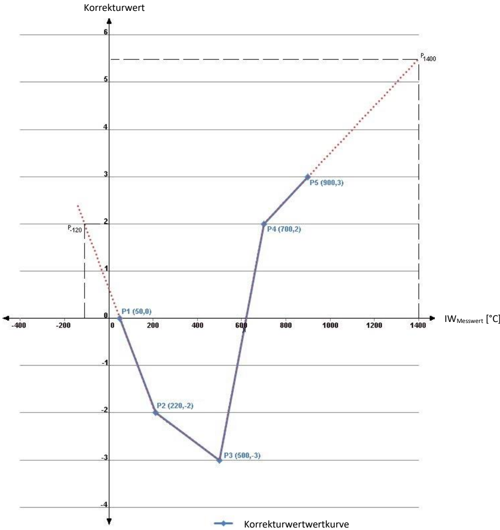
Bild 2: resultierende Korrekturwertkurve aus 5 Korrekturpunkten
