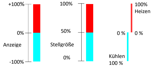
Schaltabstand = -10 % gleichzeitig Heizen und Kühlen
