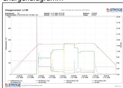
Chargendiagramm
